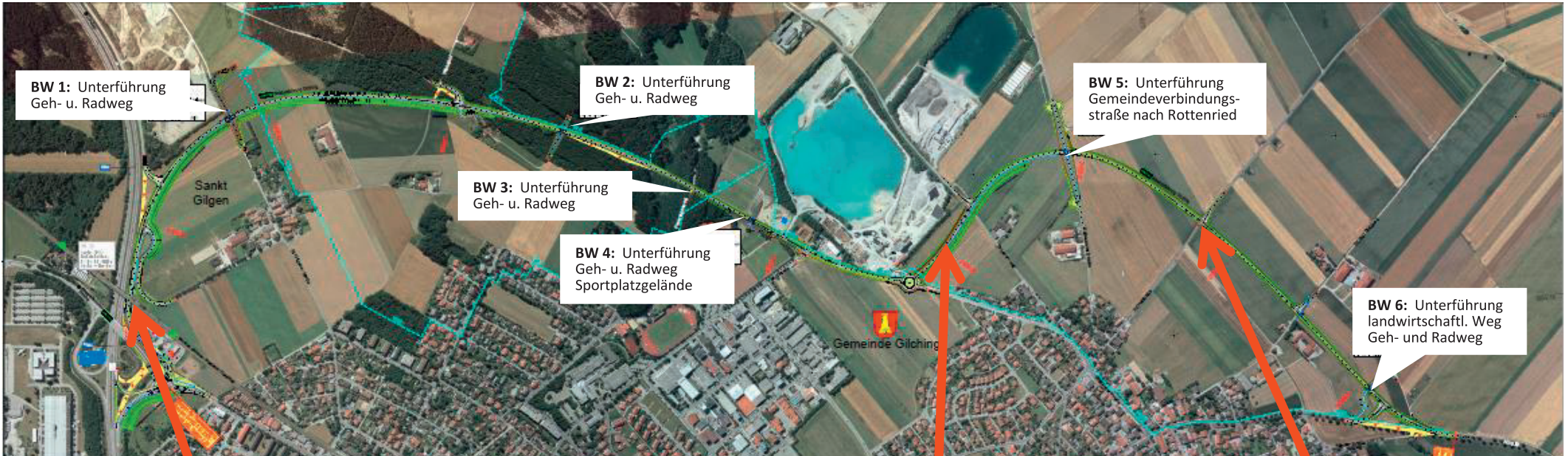
Trassenführung am Röchnerknoten ohne Erhalt des bestehenden Radwegs bis zur S-Bahn-Unterführung
